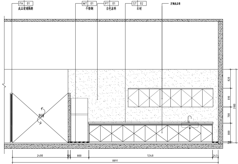
01 ELEVATION EL-01 立面图 SCALE 1: 40
