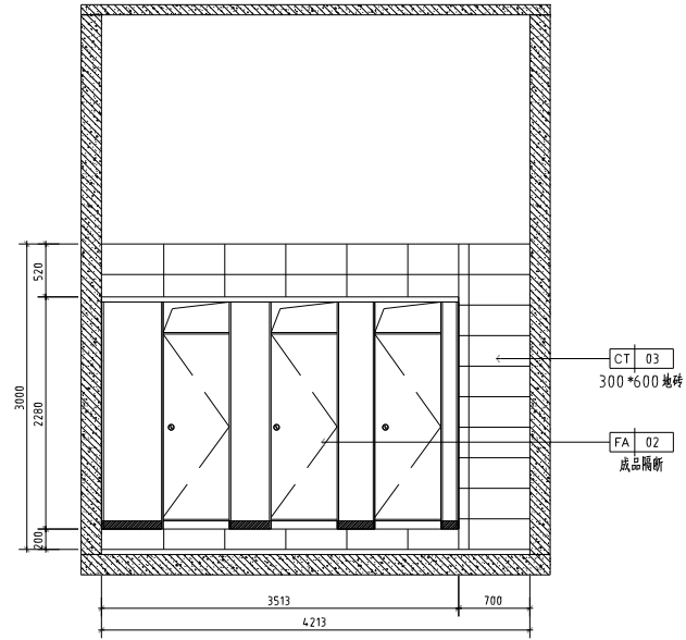
13 ELEVATION EL-01 立面图 SCALE 1: 40
