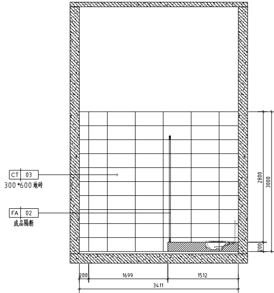
12 ELEVATION EL-01 立面图 SCALE 1: 40
