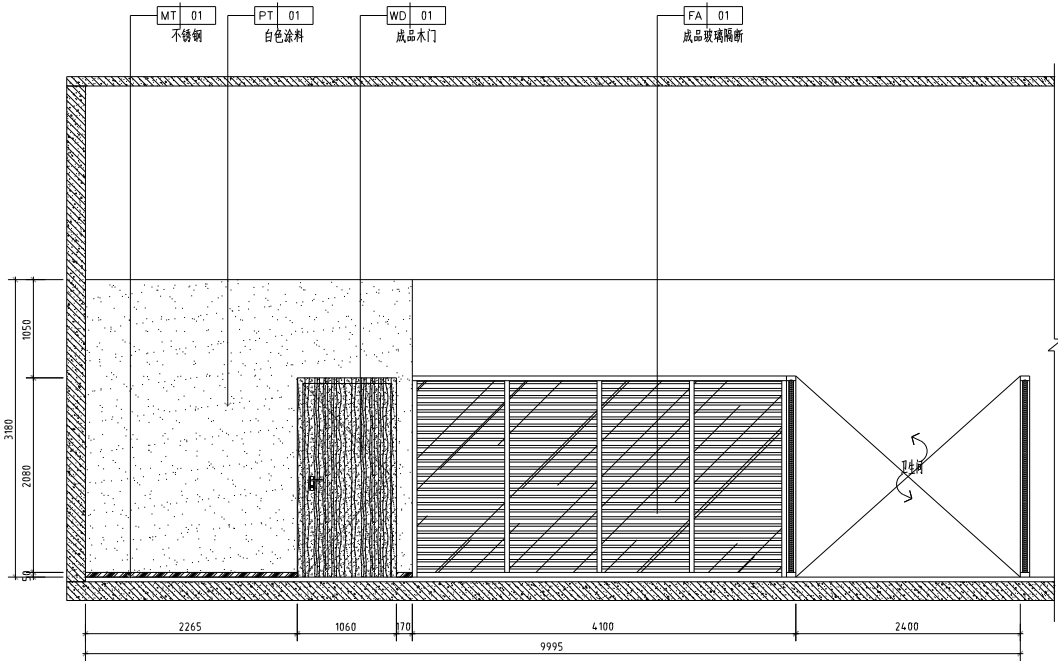
01 ELEVATION EL-01 立面图 SCALE 1: 40
