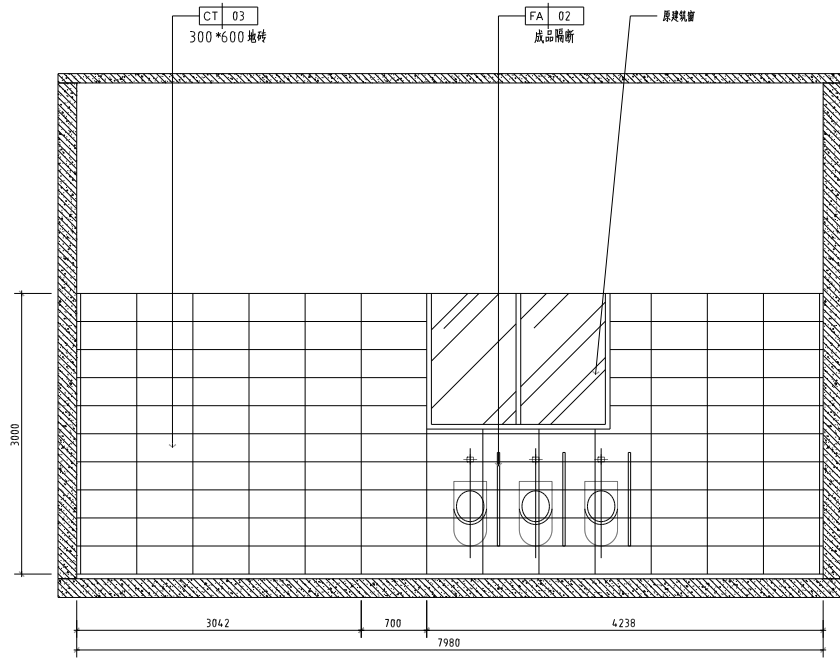
10 ELEVATION EL-01 立面图 SCALE 1: 40
