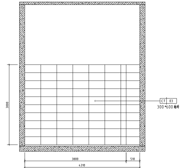
15 ELEVATION EL-01 立面图 SCALE 1: 40
