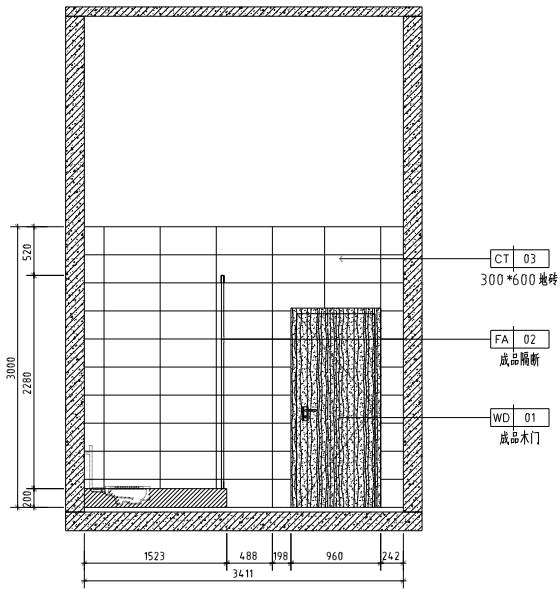
14 ELEVATION EL-01 立面图 SCALE 1: 40
