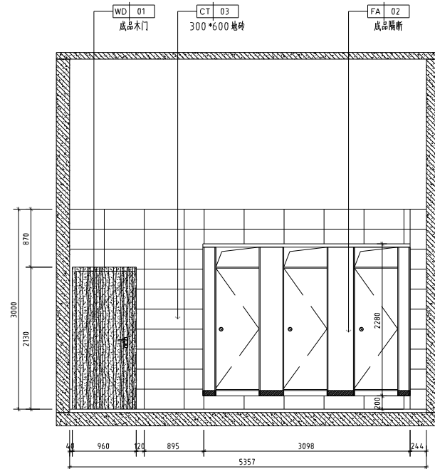
11 ELEVATION EL-01 立面图 SCALE 1: 40
