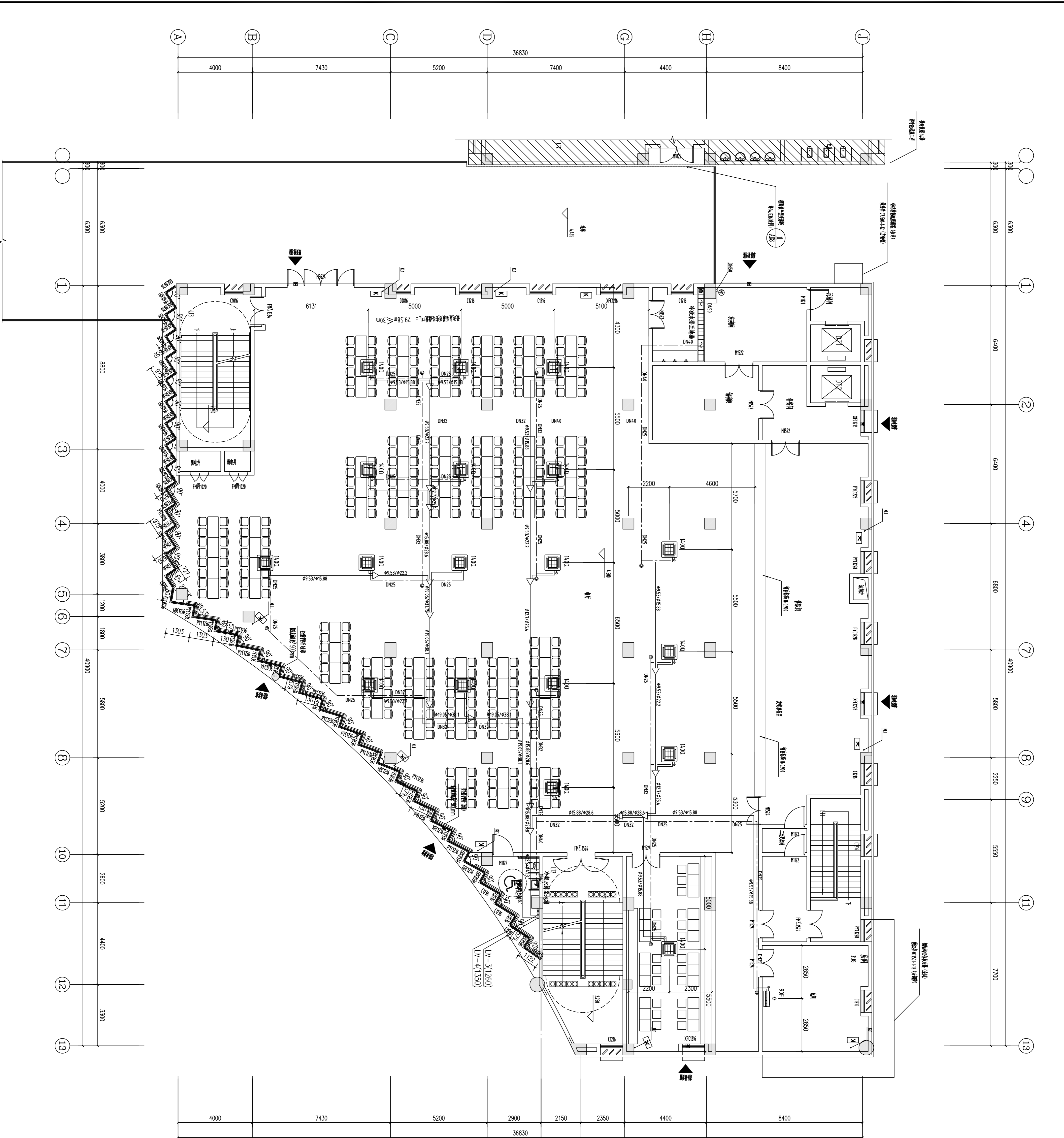
二层空调平面图 1:100
